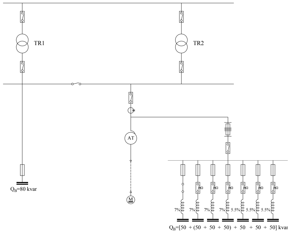
SLIKA 1: JEDNOPOLNA ŠEMA FILTERSKE KOMPENZACIJE U POGONU ŽIČARE "TORNIK"
