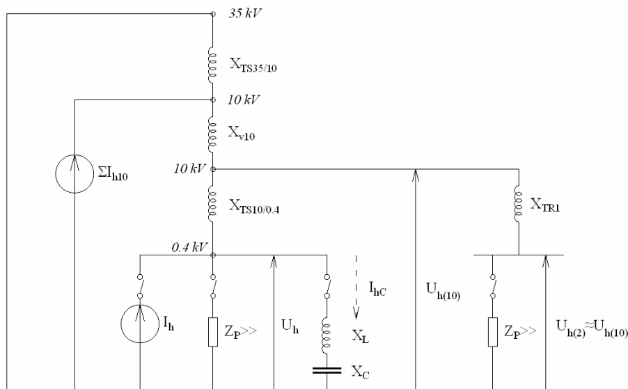
SLIKA 2: EKVIVALENTNA ŠEMA ŽIČARE "TORNIK" ZA PRORAČUN
